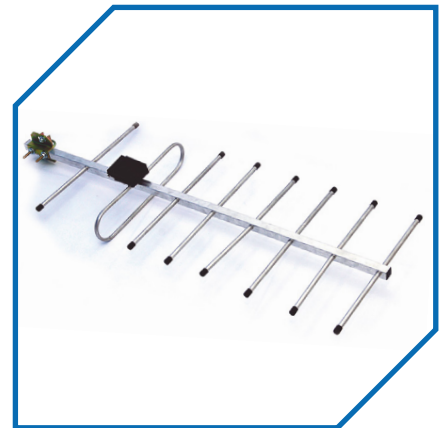
ANTENA YAGUI 7 ELEMENTOS CM 094-01 SEM CABO CM 094-02 COM CABO
