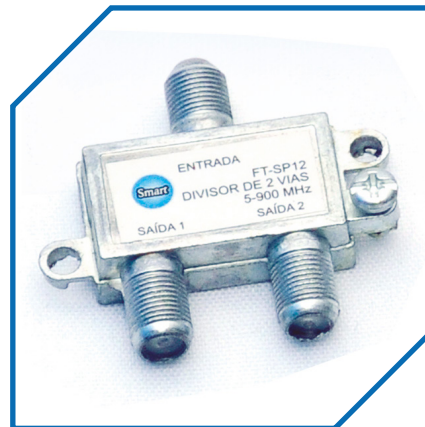
DIVISOR 1:2 VHF/UHF/CATV CM 099
